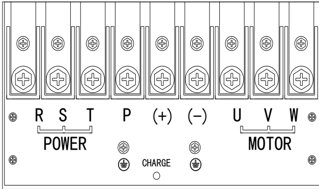
图 2-6 3PH 380V 75kW 及以上主回路端子接线
