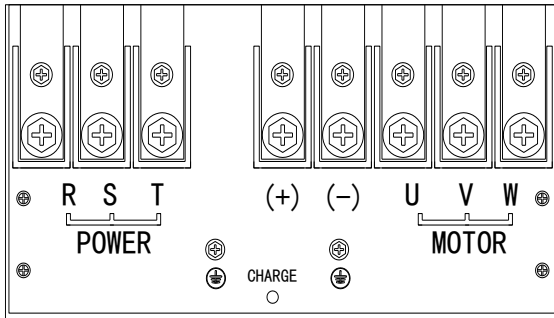
图 2-5 3PH 380V 45-55kW 主回路端子接线
