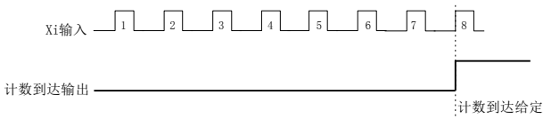
图 5-3-12 计数到达
