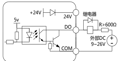
图 2-15 多功能输出端子开关量输出接线方式2
