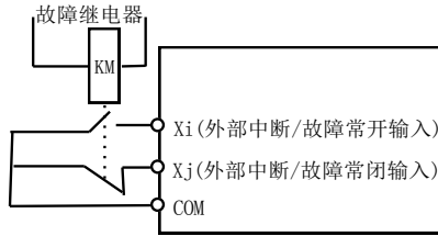
图 5-3-6 常开/常闭
