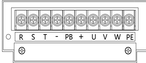
图 2-3 MT200 3PH 380V 0.75-18kW 主回路端子接线
