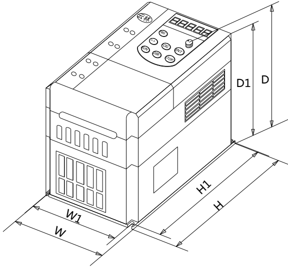
图 A4-1 外形示意图
