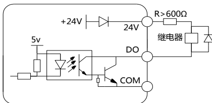
图 2-14 多功能输出端子开关量输出接线方式1
