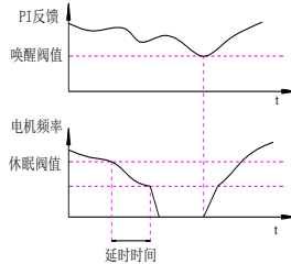
图 5-7-2 休眠和唤醒
