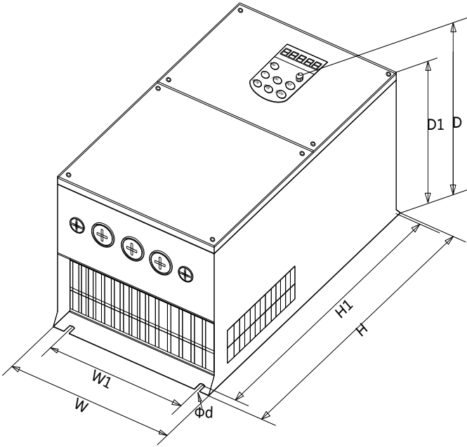
图 A4-2 外形示意图
