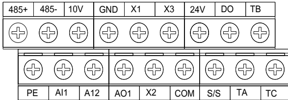
图 2-8 MT200 控制回路端子排布
