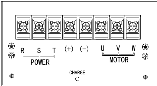
图 2-4 3PH 380V 22-37kW 主回路端子接线
