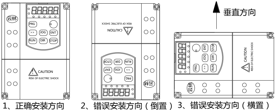
图 2-1 安装方向要求
