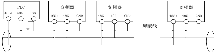
图 2-12 PLC与变频器多机通讯时推荐的接线图（变频器、电机全部良好接地）
