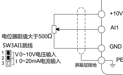
图2-9 模拟输入端子配线图
