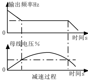
图 5-13-5 减速过程
