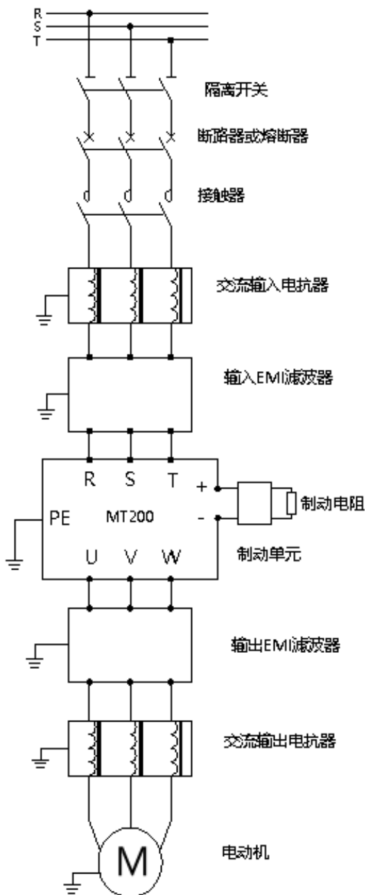
图 7-2 3018G/3022P 以上外围设备连接图 2
