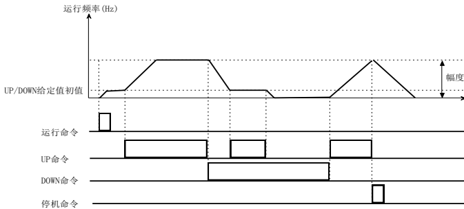
图 5-3-4 UP/DOWN 端子非组合运行
