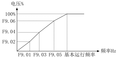
图 5-9-2 用户设定V/F曲线一般形式
