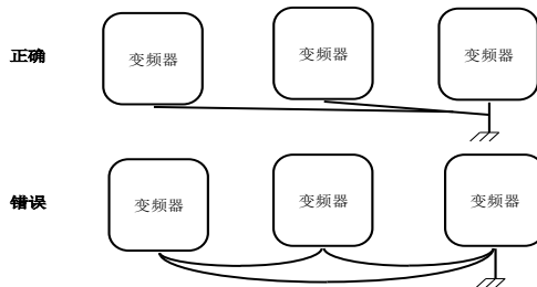
图 2-7 接地线连接方法
