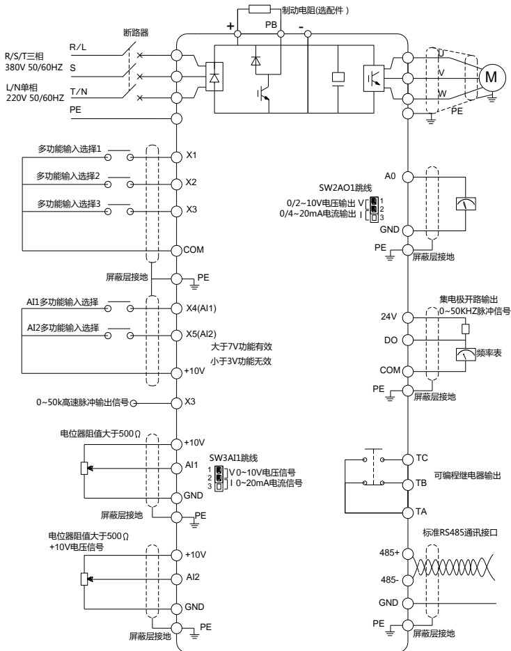
图 2-16 接线图
