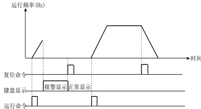
图 5-3-1 端子复位
