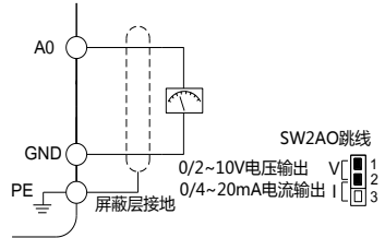
图2-10 模拟输出端子配线图
