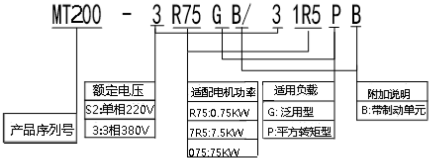
图 1-1 型号说明
