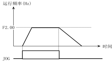
图 5-3-2 JOG运行
