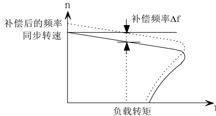
图 5-9-4 自动转差补偿
