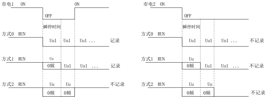
图 5-1-8 瞬停处理
