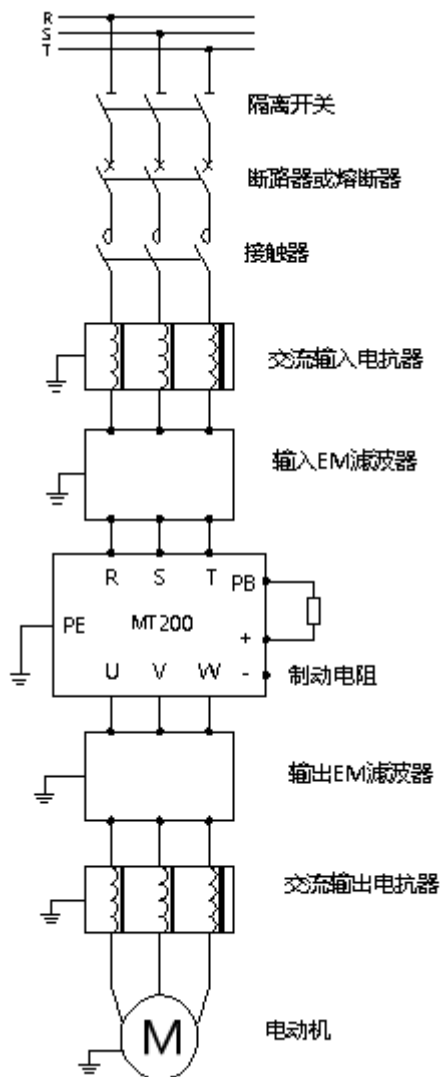
图 7-1 S3R75GB-3015GB/3018PB 外围设备连接图
