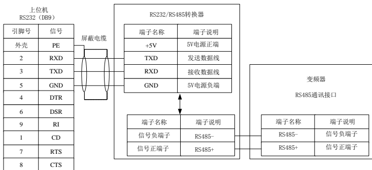
图 2-11 上位机与变频器接口接线图
