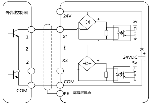
图2-13输入多功能端子配线连接图
